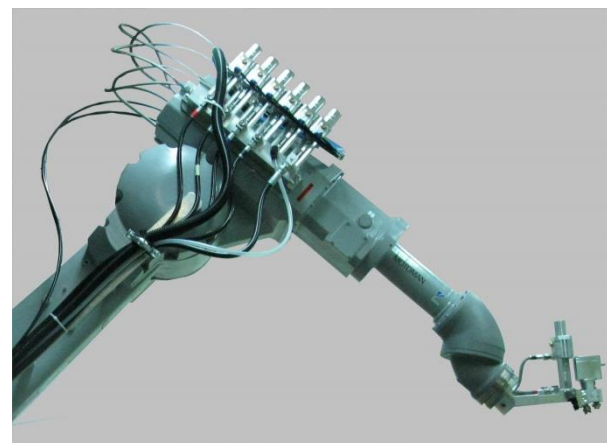
Ramię robota z głowicą natryskową i zmieniaчем kolorów
