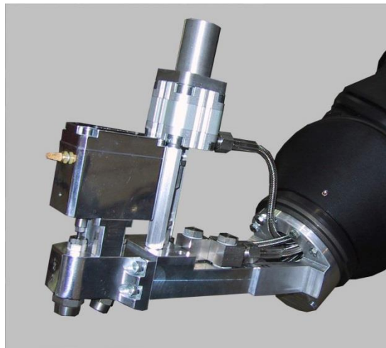
Automatyczna głowica natryskowa z zaworem zrzutowym
